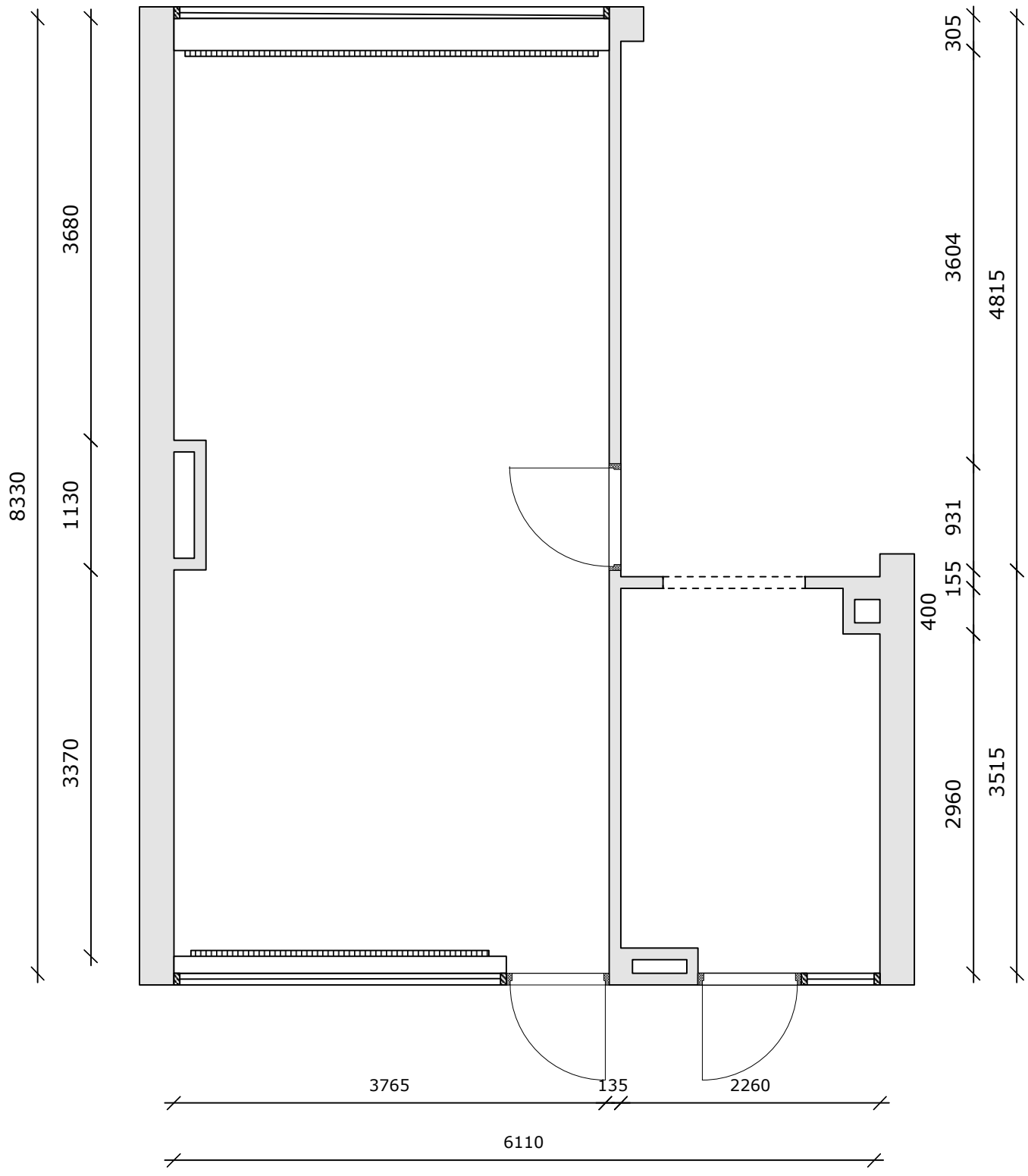
SCHETSONTWERP INDELING WOONKAMER EN KEUKEN BEGANE GROND TUSSENWONING
